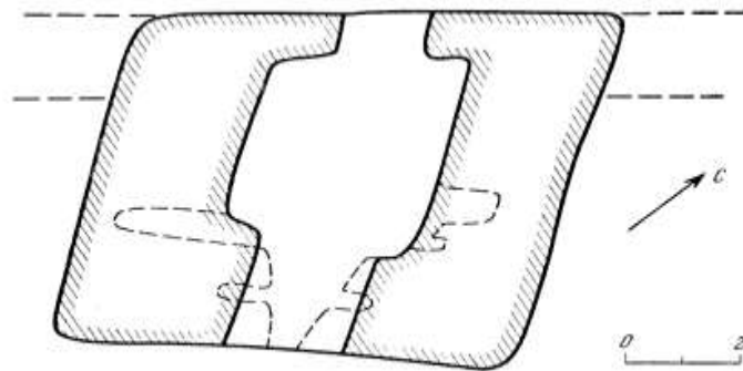
Рис. 2. Башня Ратуши. План на уровне проезда
