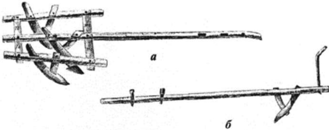
7. Рало, a — тройное рало, б — одинарное рало. Рисунок А.И.Гильденштедта. (Технологический журнал, т. I, ч. II, СПб., 1804. Приложения).
