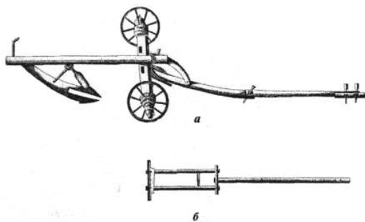
4. Соха с колесным передком и дышлом для запряжки волов (а). Упрощенный вариант с дышлом (б). (Технологический журнал, т. I, ч. II, СПб., 1804. Приложение).
