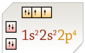
Электронное строение атома
