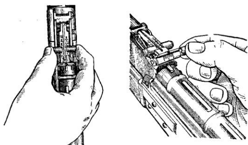
Установка прицела АК74
